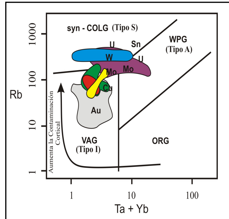
Figura N° 3.- Diagrama discriminante de granitos (Pearce, 1996), mostrando el dominio geotectónico de las diferentes provincias metalogenéticas. (ver leyenda en Figura. N°4)
