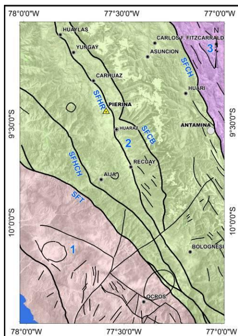
Figura. 02. Sistemas de fallas y dominios tectónicos
