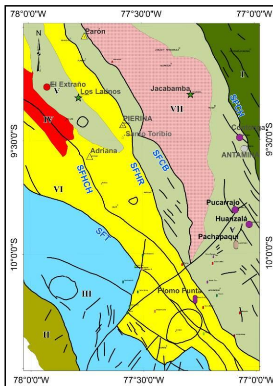
Figura 03.- Metalogénica del área de estudio
