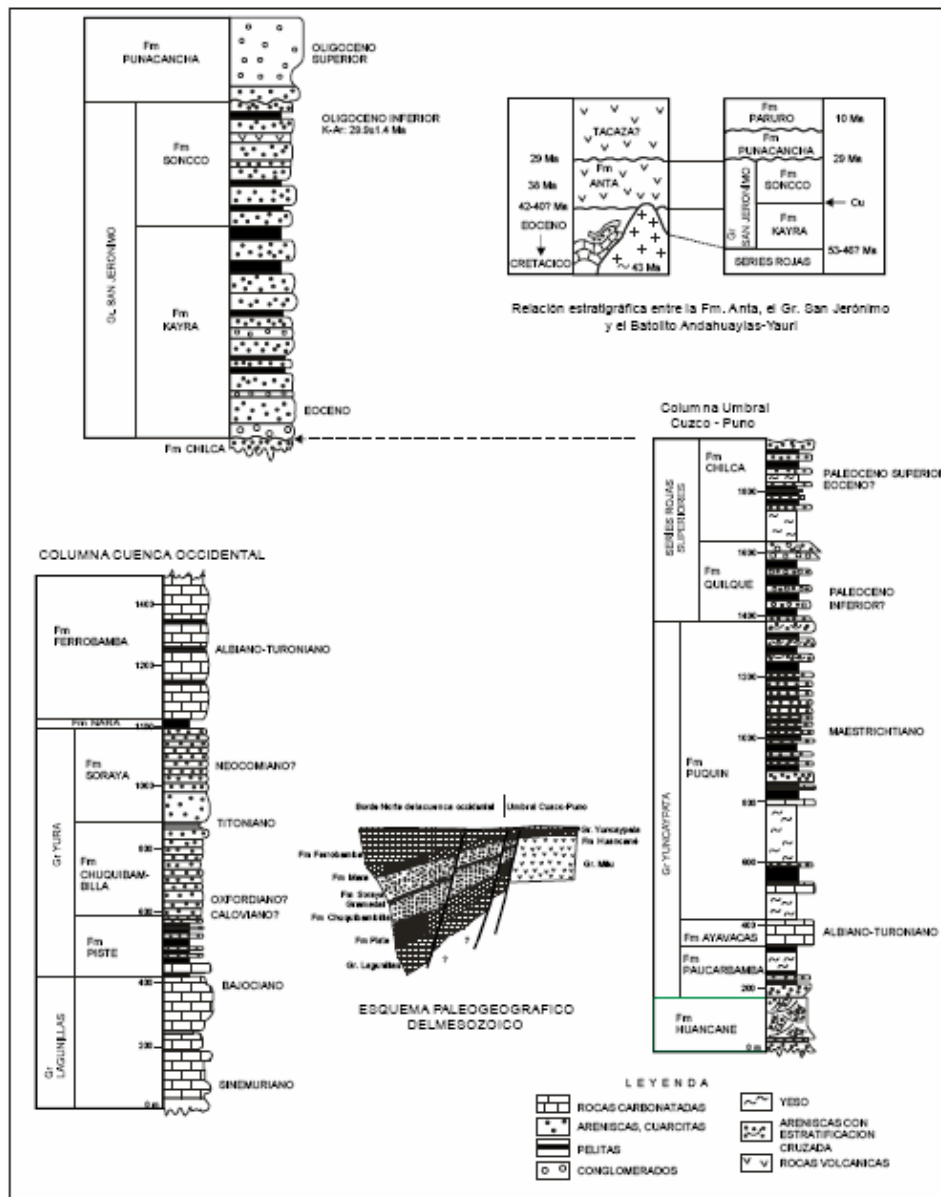
Fig. 2.1.- Regional stratigraphic columns (Carlotto et al., 1996, 1999).
