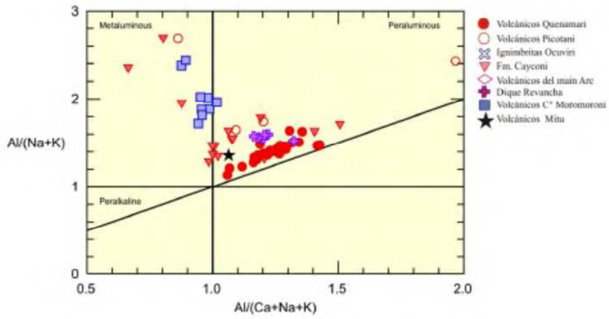
Fig. 16.- Diagrama de Saturación de Alúmina (Manjar & Piccoli, 1989),
