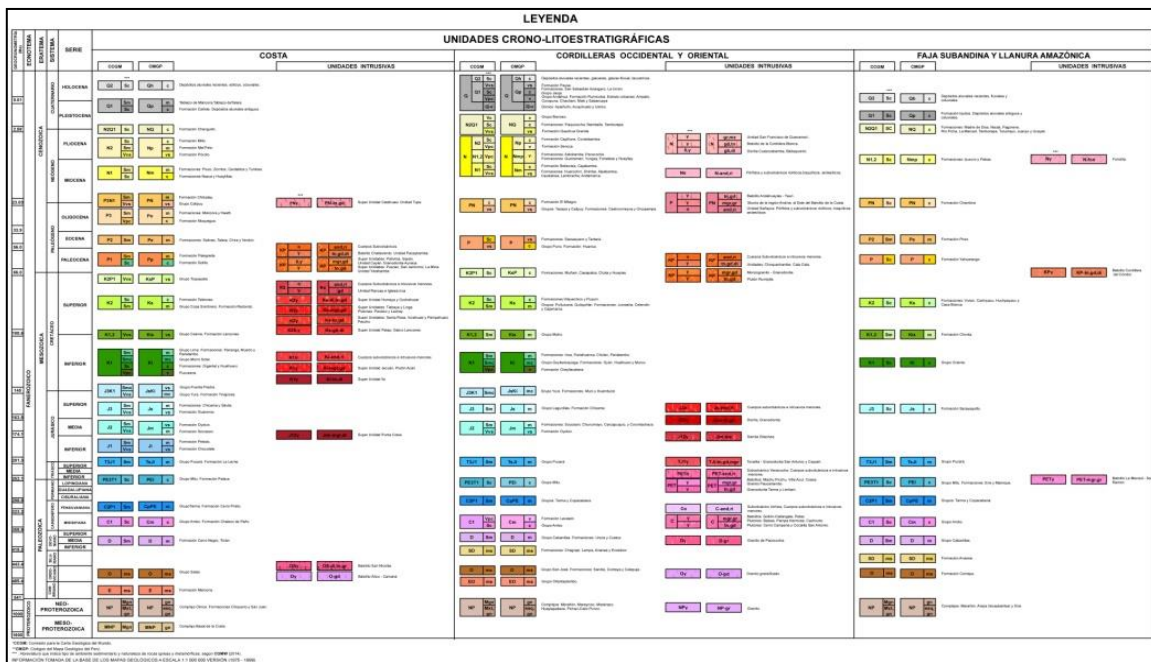
Figura 2. Leyenda Geológica de Unidades Crono-Litoestratigraficas de la nueva versión digital estandarizada del Mapa Geológico del Perú a escala 1:1'000,000.
